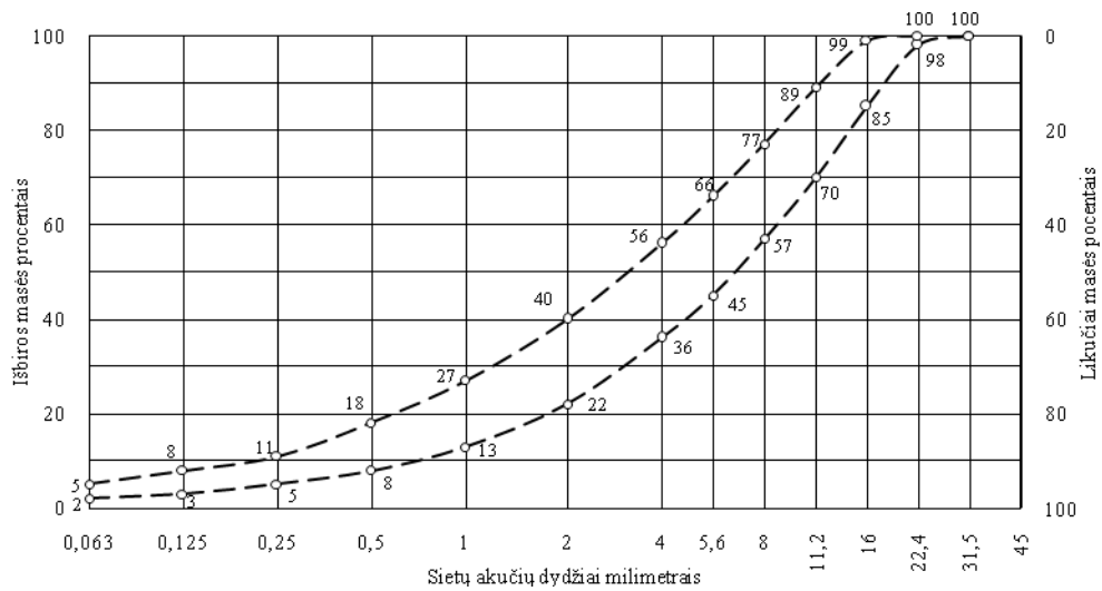
1 pav. Paviršiaus apdaro mineralinių medžiagų mišinio 0/16 granulimetrinės sudėties ribos
