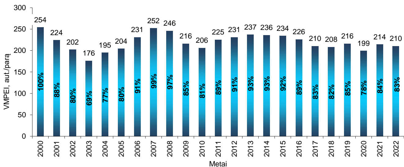
Krovinio transporto vidutinio metinio paros eismo intensyvumo kitimas krašto keliuose nuo 2000-ųjų metų
