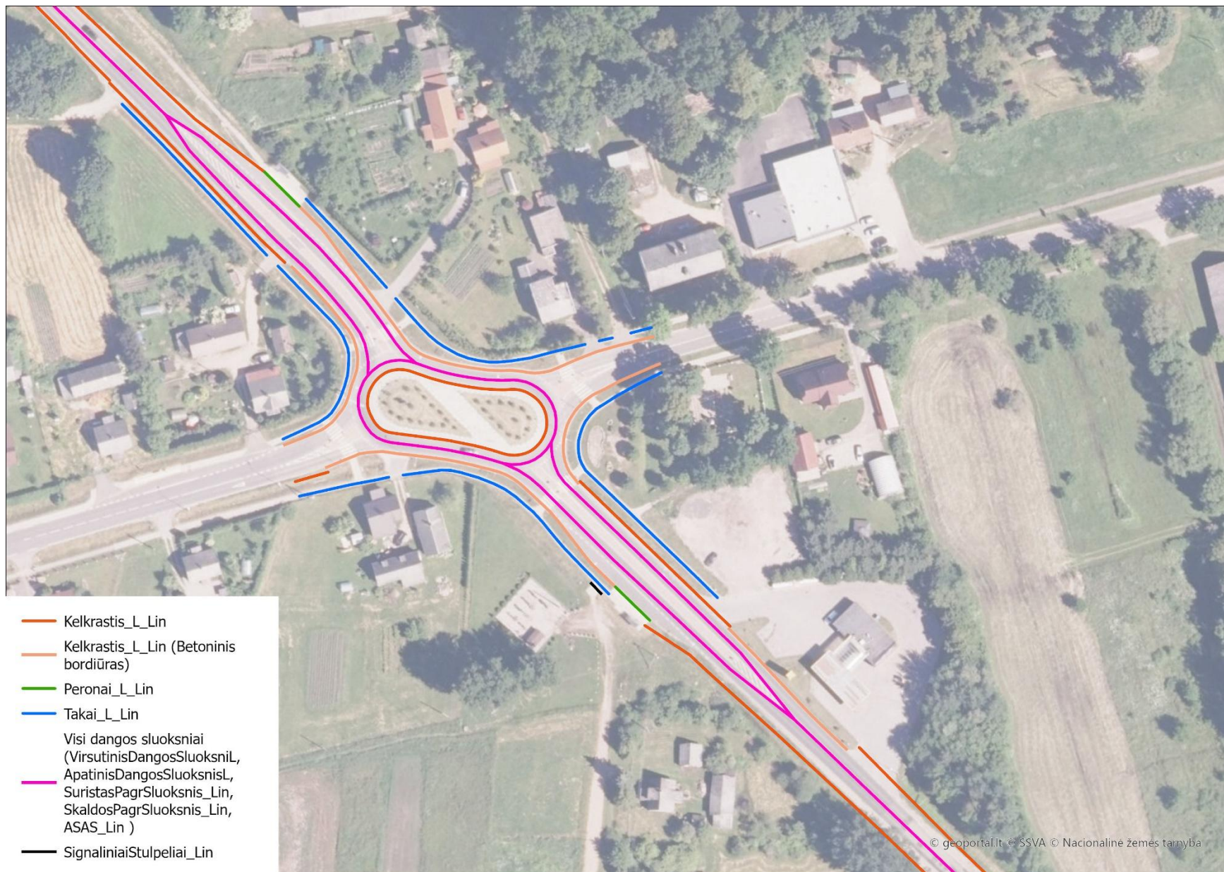
4 iliustracija. Kelio linijiniai elementai
