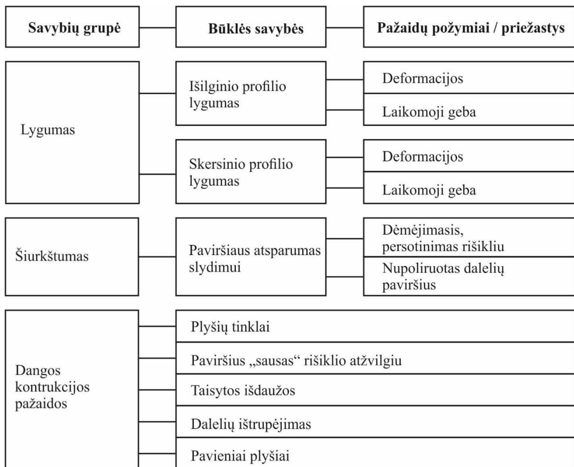
1 pav. Asfalto dangos savybių grupių, savybių ir pažaidų požymių priklausomybės schema
