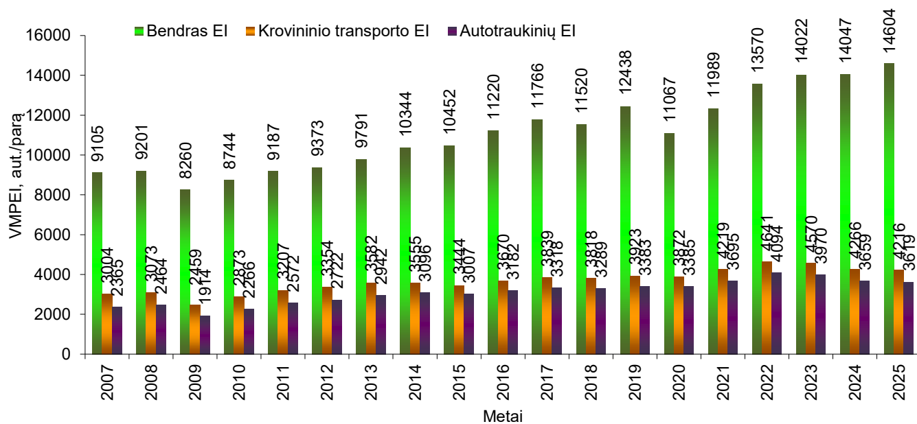
Vidutinio metinio paros eismo intensyvumo kitimas transporto koridoriuje Via Baltica nuo 2007-ųjų metų
