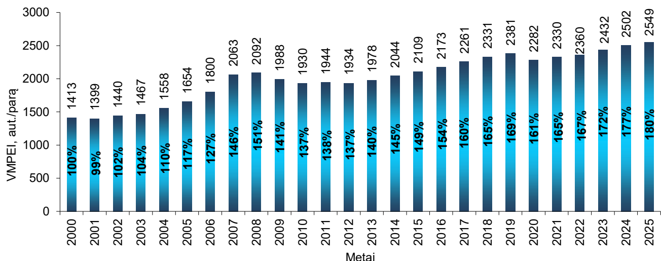
Vidutinio metinio paros eismo intensyvumo kitimas krašto keliuose nuo 2000-ųjų metų
