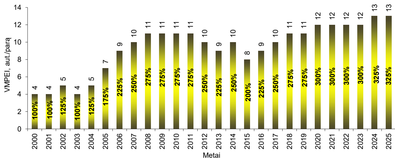
Autotraukinių (krova >12 t) vidutinio metinio paros eismo intensyvumo kitimas rajoniniuose keliuose nuo 2000-ųjų metų
